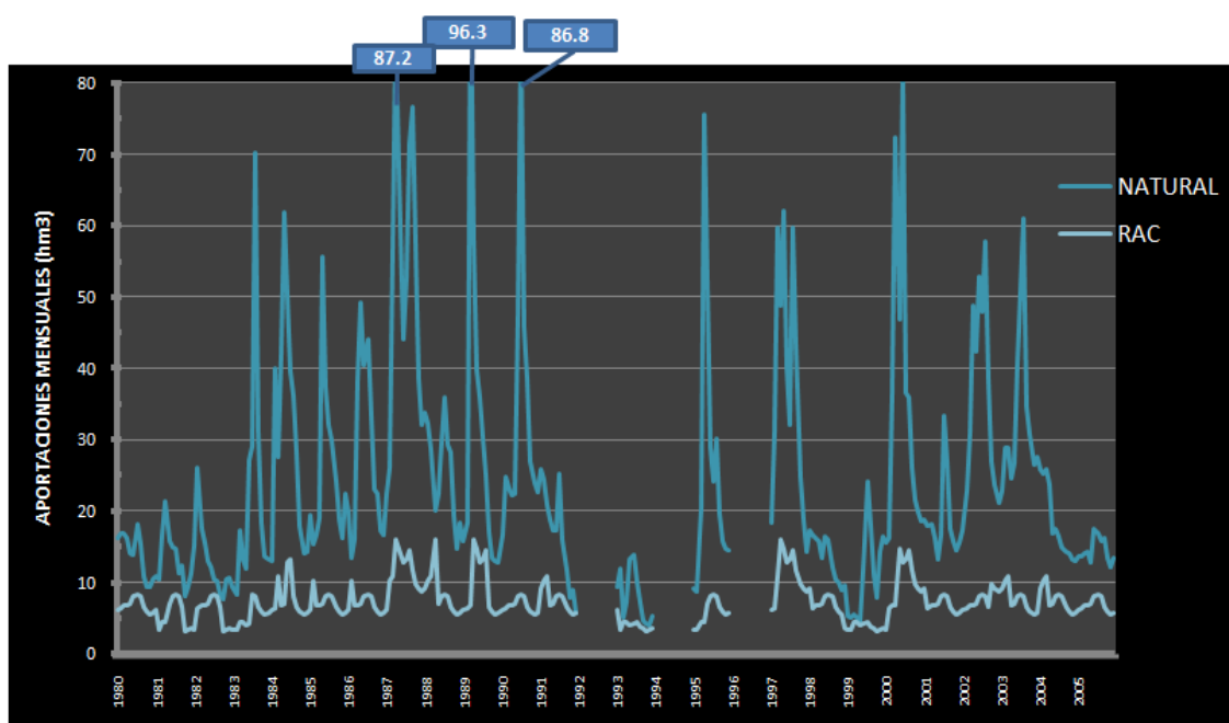
Figura nº13. Simulación de las aportaciones mensuales para un escenario RAC ( m=2 ; K=0,41 ). Río Cabriel, en el embalse de Contreras.
