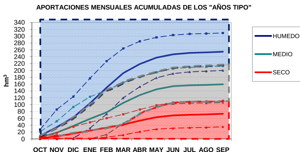
Figura nº11. Aplicación de criterios para la obtención de la gráfica para la discriminación del tipo de mes -húmedo, medio o seco-, a partir de los intervalos de confianza (90%) de las aportaciones mensuales acumuladas en RN. Río Jarama en El Vado.
