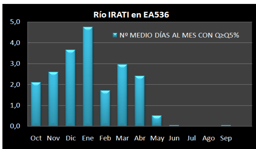
Figura nº5. Información de estacionalidad y duración de avenidas en RN ofrecida como gráfico en el informe nº4 de IAHRIS. Río Irati en EA 536.
