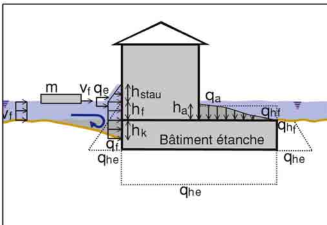
Figure 5.6 : Crues : inondation dynamique avec érosion et alluvionnement (suivant VKF-AEAI)
