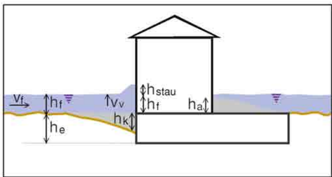
Figure 5.2 : Crues : notations (suivant VKF-AEAI)
