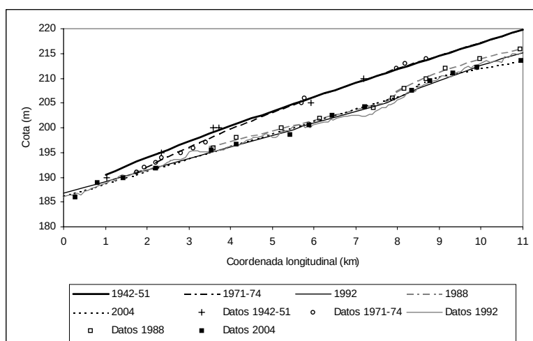
Figura 1. Incisión lineal en el bajo Gállego, tramo de Montaña (Martín Vide y Ferrer, 2005)
