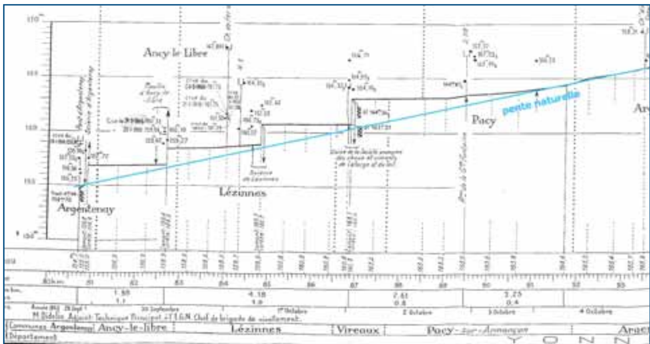
Figure 34 : Exemple de profil en long fortement altéré par la présence de seuils. L'Armançon (89) (source : IGN). ≡
