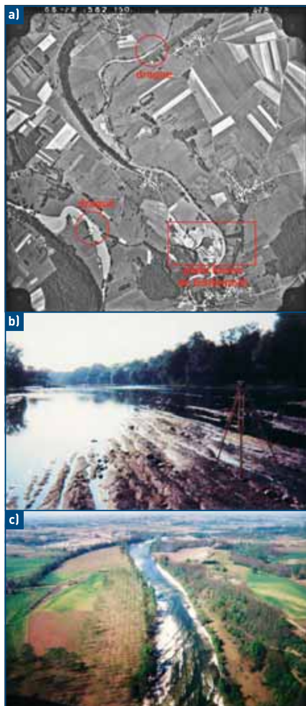
Figure 37 : a) Extractions alluvionnaires en lit mineur par drague flottante. Noter les sur-élargissements liés à l'extraction en profondeur et en largeur. b) Résultats : incision généralisée du lit et absence d'alluvions sur le fond du lit mineur (la photo de gauche montre les traces de « dents » des pelleteuses dans les marnes). c) On exploitait souvent jusqu'au substratum avec l'apparition de la roche mère sur de nombreux cours d'eau. ≡
