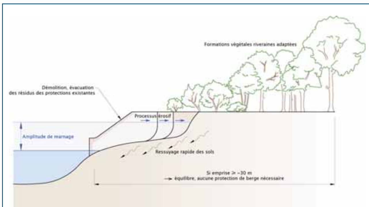
Figure 51 : Si l'emprise est élargie, aucune protection de berge n'est nécessaire en présence de contraintes de marée. ≈
