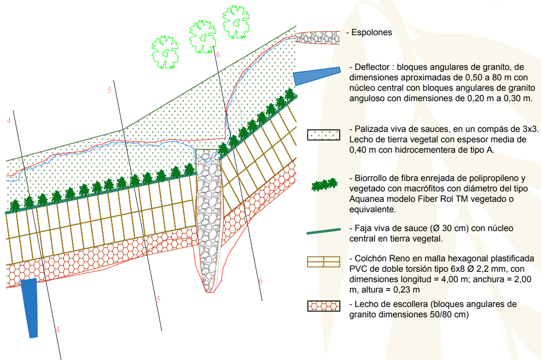
Figura 2. Parte de una planta general de una intervención propuesta conteniendo los perfiles 4, 5 y 6.
