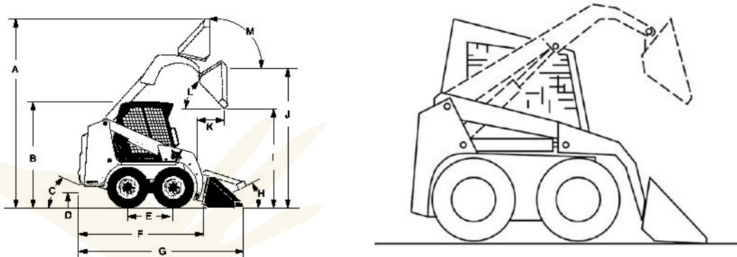
Figura 1. a) Representación del área de trabajo de una máquina mixta, parte frontal pala cargadora y retropala trasera. Dibujo: MF Industrial. b) Dibujo de una minicargadora. Dibujo: Bobcat.
