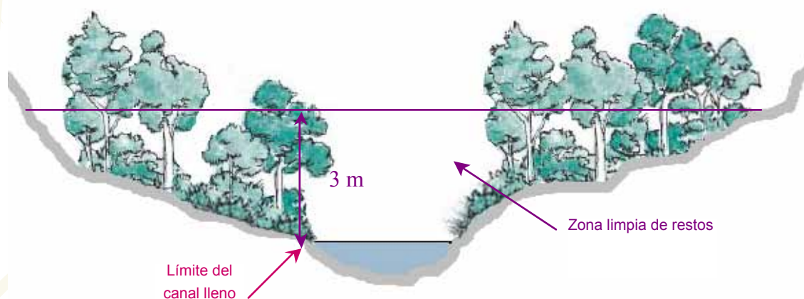
Figura 18. La zona situada a una cota inferior a 3 m sobre el canal lleno estará limpia de restos de corta o desbroce. Dibujo: Roser Casas.
