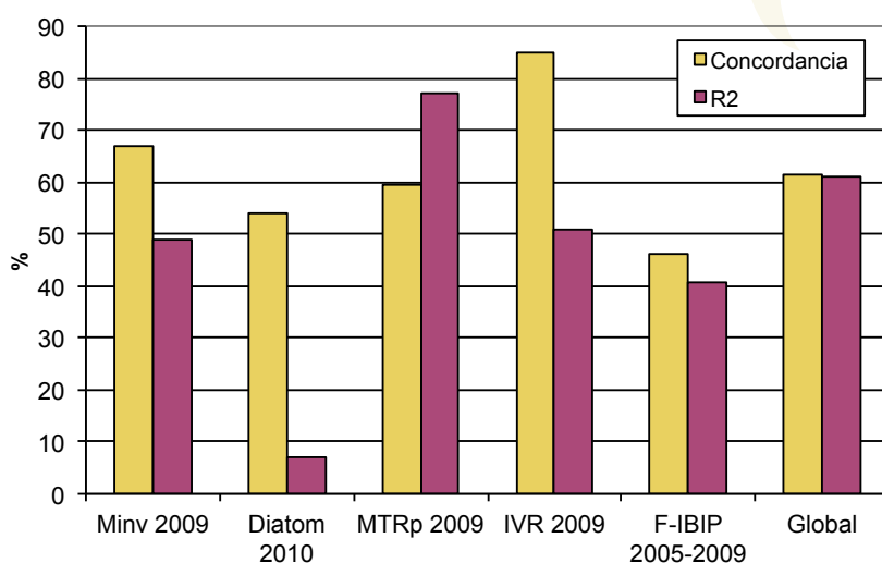
Figura 17. Representación de la concordancia y el coeficiente de determinación para los indicadores de calidad biológica. A nivel global se representa la concordancia a través de la media de las concordancias de los elementos de calidad y el coeficiente de determinación del ajuste de la media de los elementos de calidad biológica. Intervalo de confianza del 90%.
