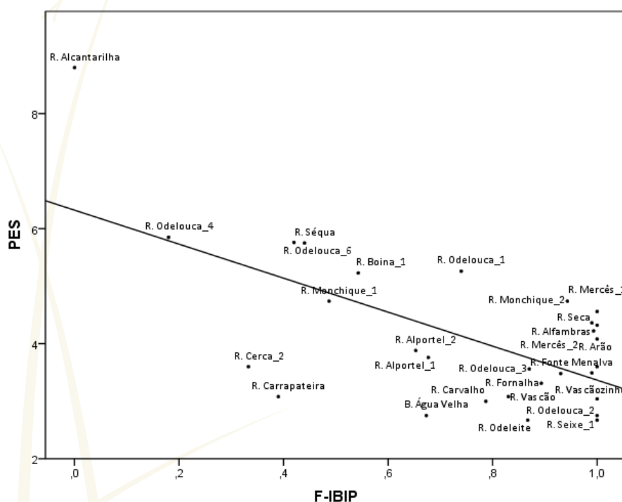
Figura 16. Representación del ajuste lineal del F-IBIP con la PES. R^2 = 0,405 , PES = 6,322 - 2,956 * F-IBIP .
