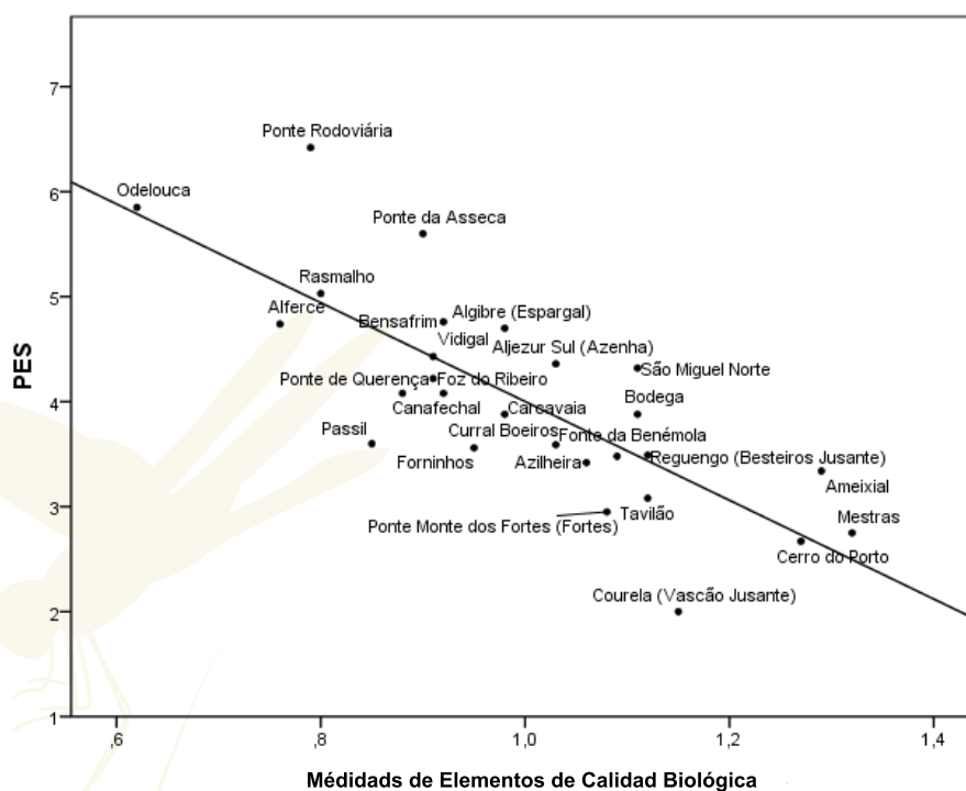
Figura 18. Representación lineal en un intervalo de confianza del 90% de las medias de los indicadores de calidad biológica con la PES. R^2 = 0,61 PES = 9,389 - 5,327 * \text{Calidad biológica} .
