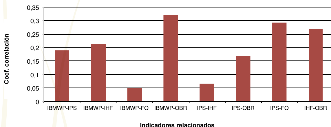
Figura 2. Correlación entre todos los indicadores analizados en la serie histórica 2005-2009.
