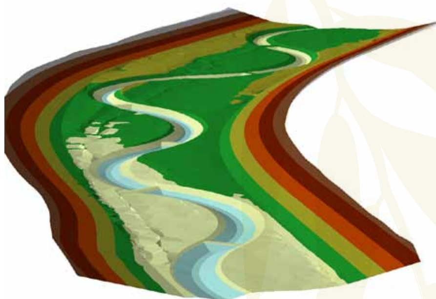
Figura 2. Modelo digital del terreno que ejemplifica una de las hipótesis testadas para el modelo hidráulico River 2D: introducción de islas en un segmento artificialmente meandrizado.
