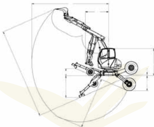
Figura 3. a) Representación del área de trabajo de retroaraña. Dibujo: Menzi Muk. b) Retroaraña trabajando en un río.
