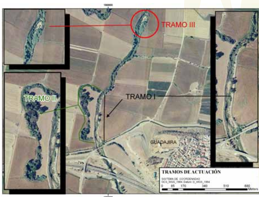
Figura 2. Definición concreta de los tramos a restaurar en el río Guadajira (Badajoz).
