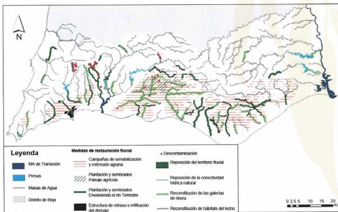
Figura 1. Representación de la carta de optimización de las medidas de acción de restauración.
