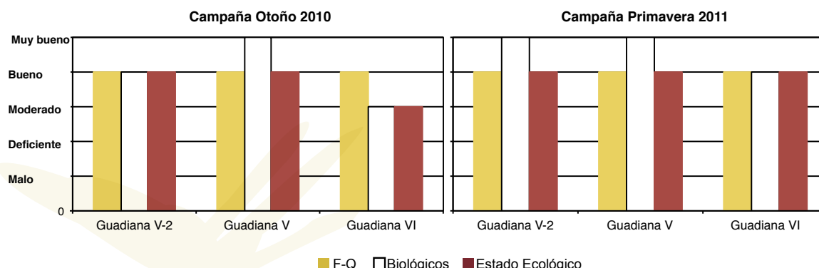
Figura 9. Gráfico de la calidad ecológica de cada uno de los elementos para la tipología 108.
