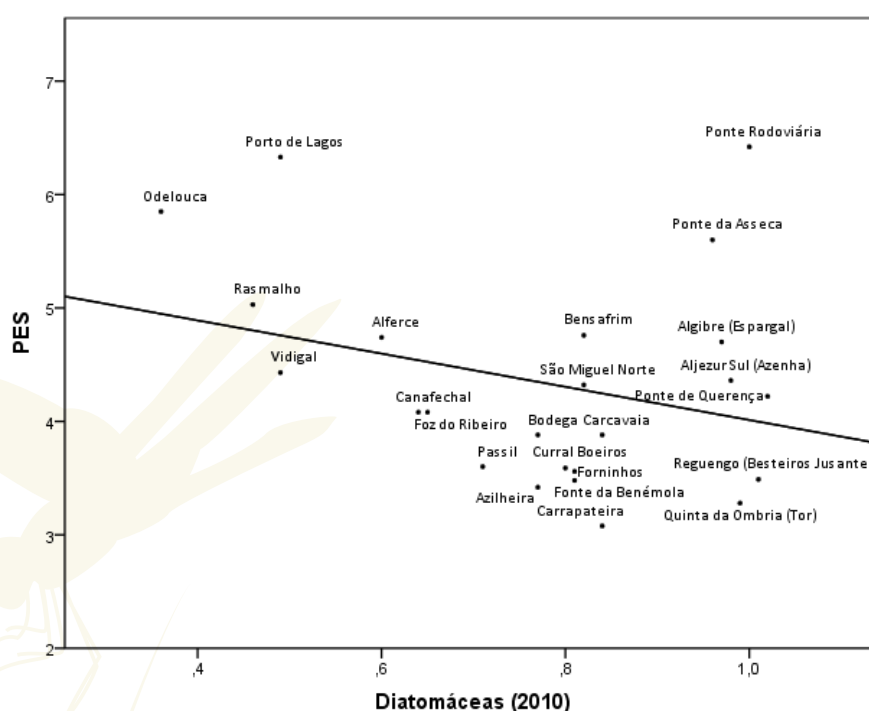
Figura 14. Representación del ajuste lineal de las diatomeas en el período de 2010 con la PES. R^2 = 0,089 , PES = 5,4754 - 1,4632 * Diatomáceas .
