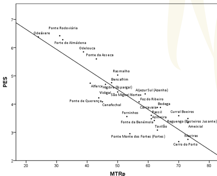
Figura 15. Representación del ajuste lineal del MTR p en el período de 2009 con la PES en un intervalo de confianza del 90%. R^2=0,776 PES = 8,0667 - 0,071 * MTR_p .
