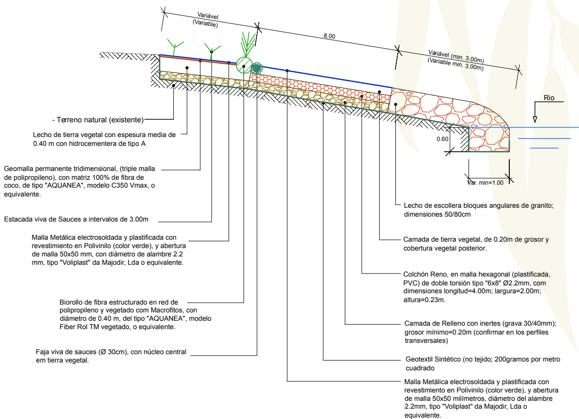
Figura 3. "Perfil tipo" con especificaciones de los materiales utilizados.
