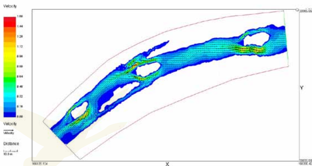
Figura 3. Simulación del canal con inclusión de islas.
