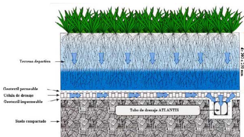
Perfil de un campo deportivo
